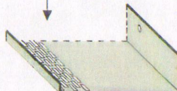
GELOCHTES SOCKELPROFIL
